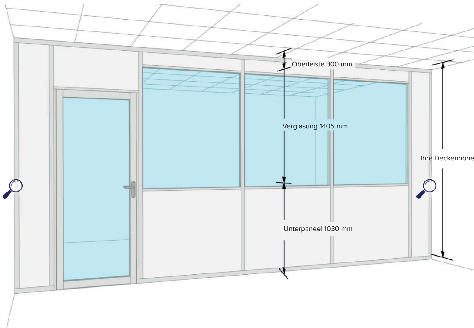
Befestigung der Bürotrennwand unter der Decke
