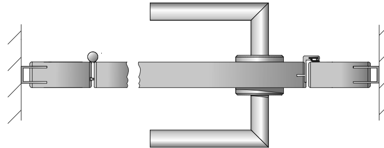
2 Plan de coupe de la façade avec poignée de porte
