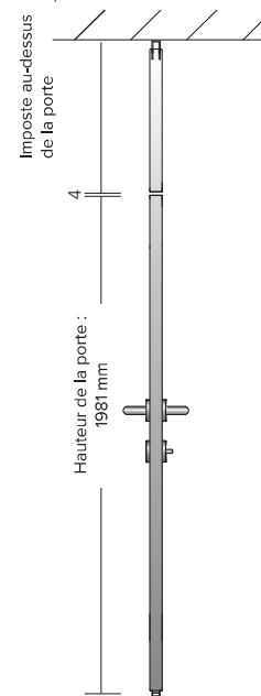
3 Plan de coupe de la hauteur
