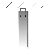
5 Raccordement au mur avec un profilé en U comme joint caché
