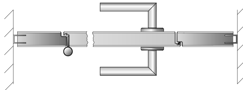
Plan de coupe de la façade avec poignée de porte
