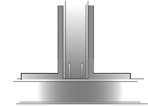
3 Connexion façade - paroi de séparation
