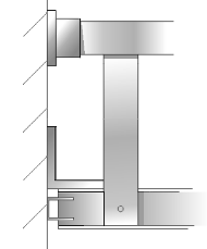
5 Connexion mur - façade
