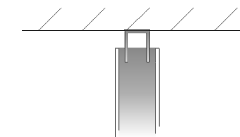
5 Raccordement au mur avec un joint creux
