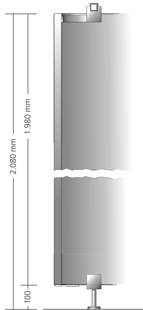
1 Plan de coupe connexion façade - paroi de séparation
