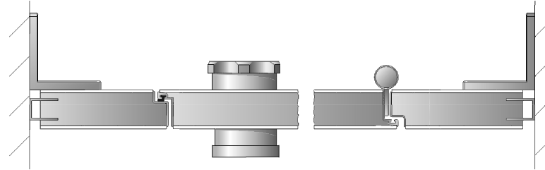
2 Plan de coupe de la façade avec bouton de porte - Charnières auto fermantes en aluminium
