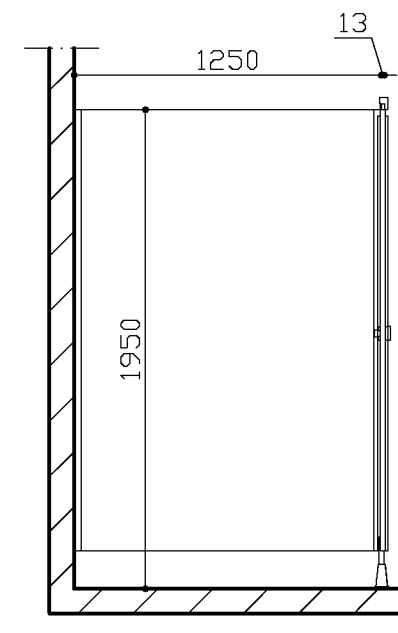
ZIJAANZICHT VOOR- EN SCHEIDINGSWAND
