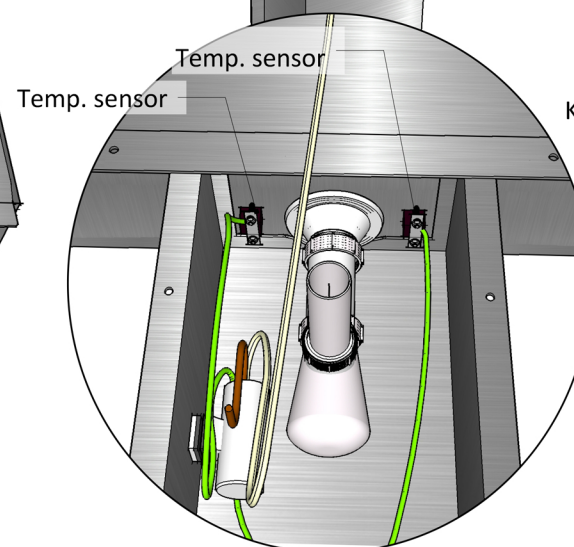
aansturing ventiel
